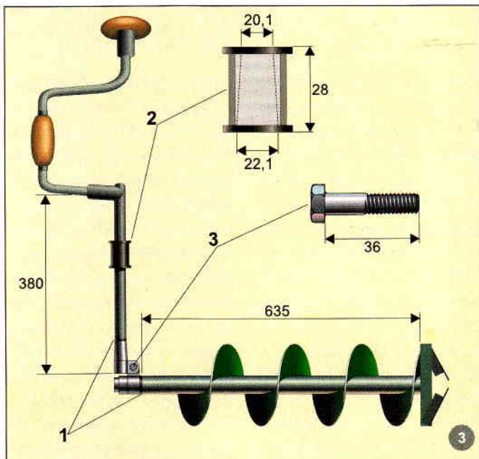
3. Переделка соединительного узла ледобура "Ленинградский": 1 – соединительный болт М8; 2 – места электросварки; 3 – свободно скользящая фиксирующая муфта.
