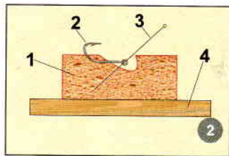
2. Форма для отливки мормышек “Уральская”: 1 – хлеб; 2 – булавка; 3 – крючок; 4 – деревянная подставка.
